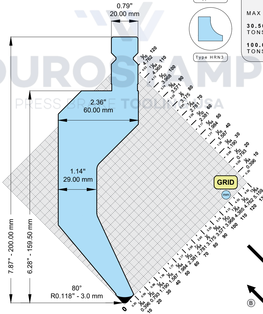
Type SF3
